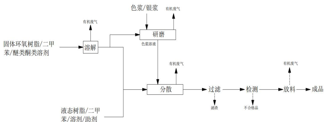
图 3 生产工艺流程图
